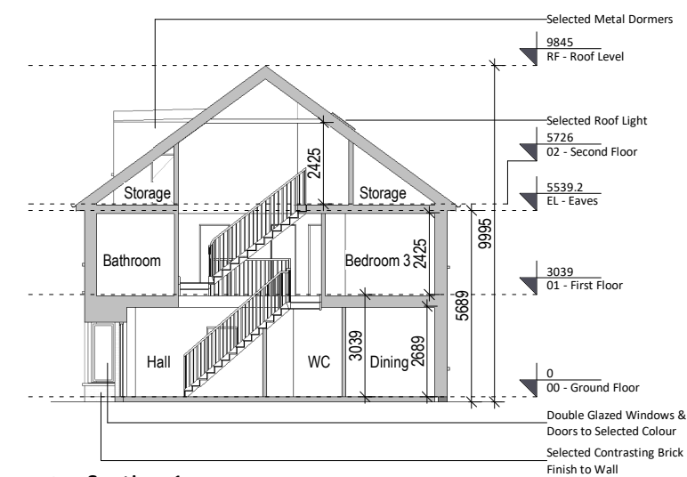
8 Section 1 1 : 200
